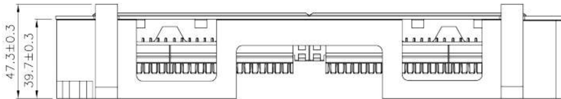
CAT.5E 6 PORT PCB MODULE
